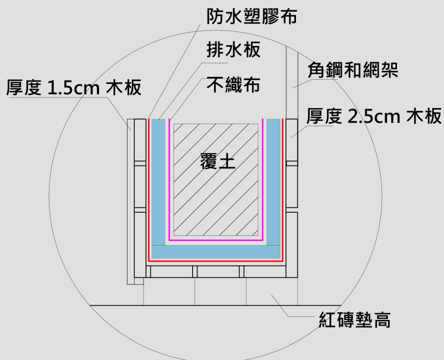
花台剖面圖
